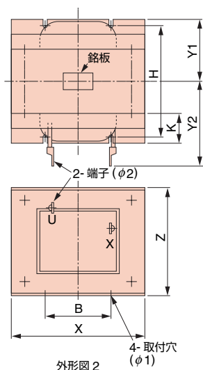
外形図 2
