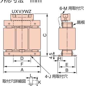
外形図 1
