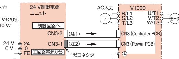
接続図
