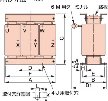
外形図 1
